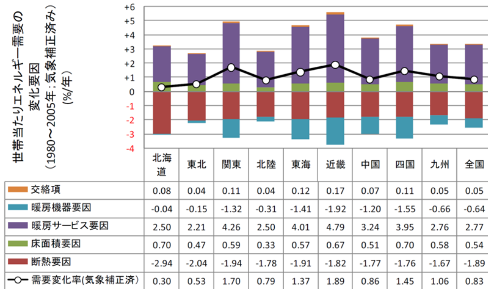
図 19 技術・ライフスタイル・床面積要因が世帯当たり暖房エネルギー需要(気象補正済)に与えた影響度
