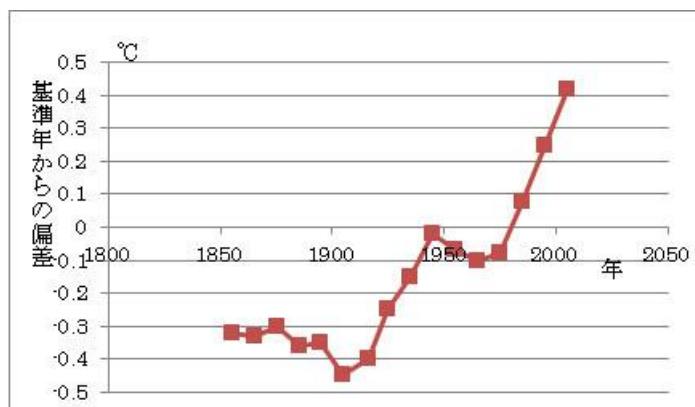
図 2-4 世界の平均地上気温の経年変化
