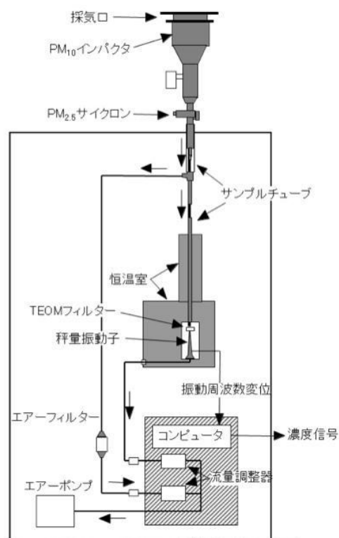
図4 TEOMによるPM 2.5 連続測定装置の概略 (EPA/625/R-96/010aを参考に作成)
