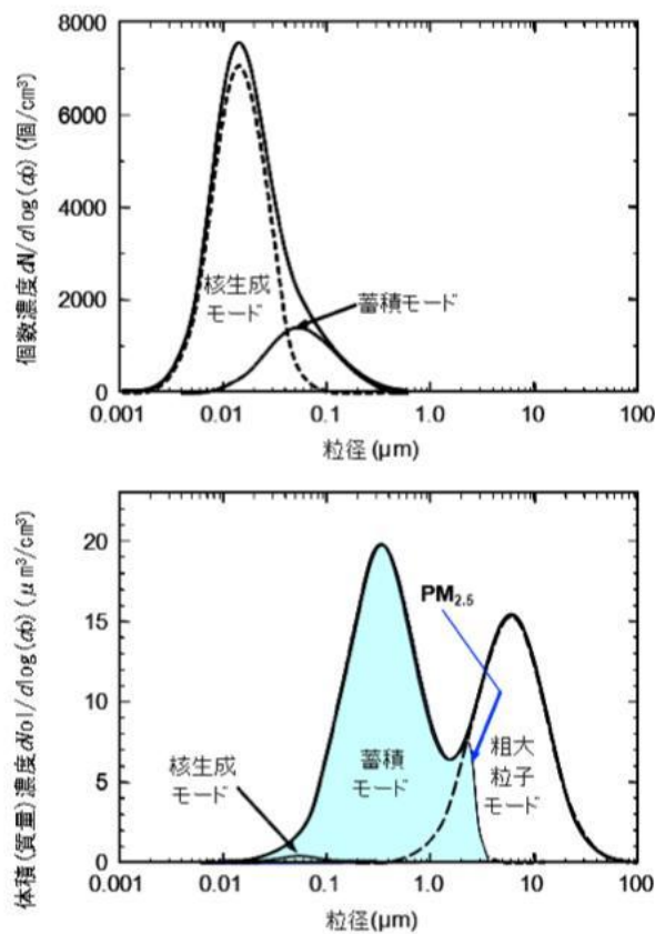
図2 都市大気粒子の粒径分布
