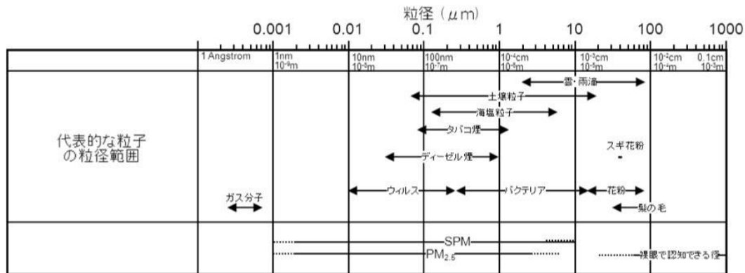
図1 代表的な粒子状物質の粒径
