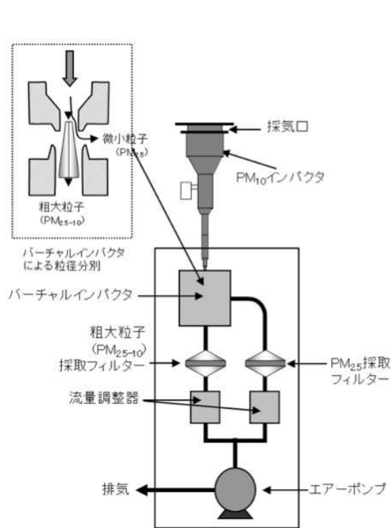
図3 FRMサンプラー装置の概略例
