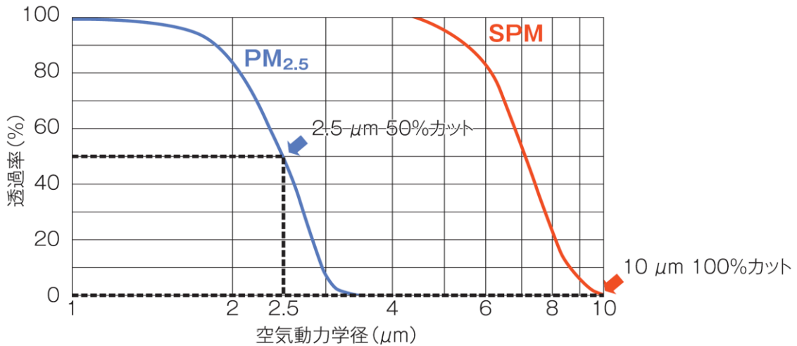
図1 PM 2.5 とSPMの透過率曲線
